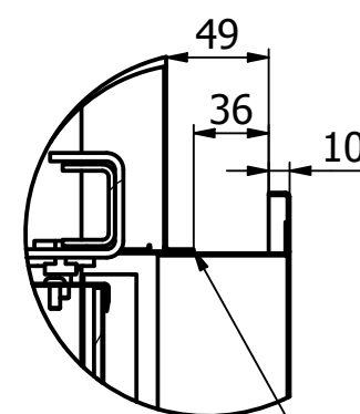
C ( 1 : 4 )
