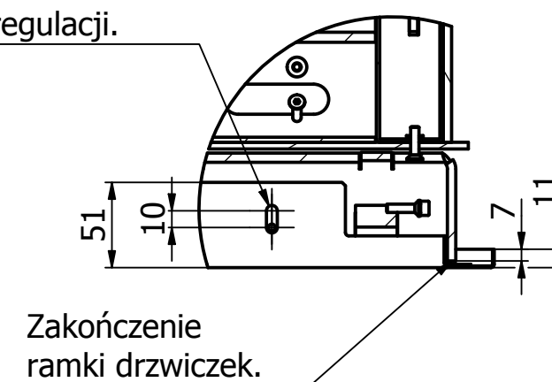
C ( 1 : 4 )
