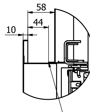
A ( 1 : 4 )
