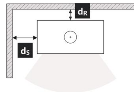
Рис. 3 Расстояние от невоспламеняющихся материалов
