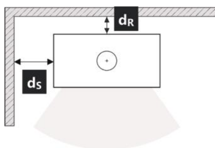
Obr. 3 Bezpečnostní odstupy od nehořlavých materiálů
