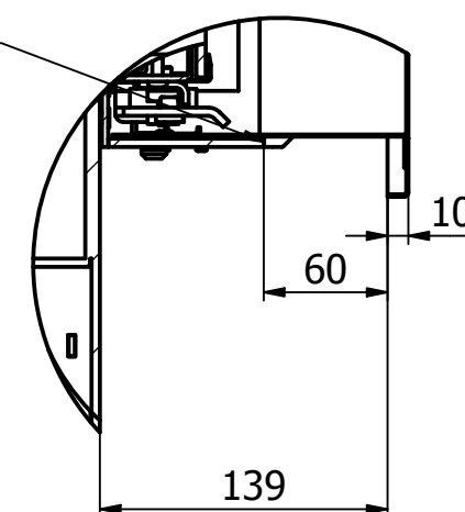
D ( 1 : 4 )
