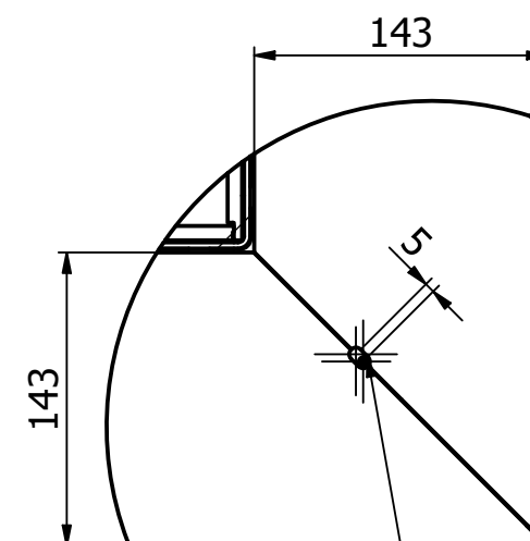
E ( 1 : 4 )
