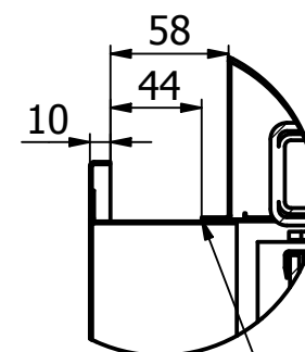
A ( 1 : 4 )
