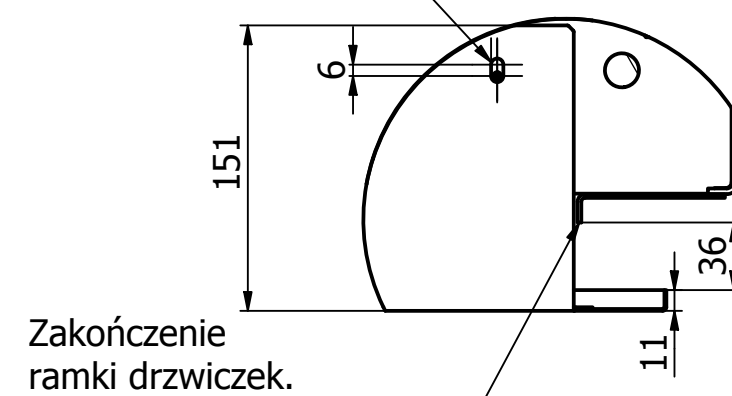
C ( 1 : 4 )
