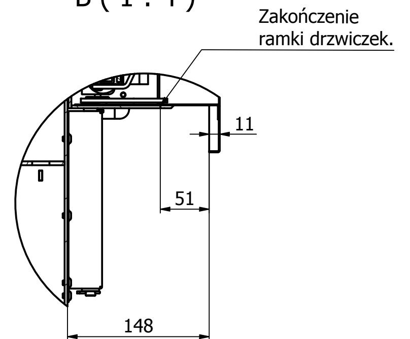
B ( 1 : 4 )
