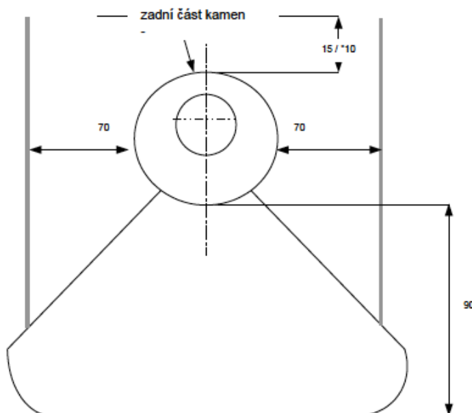
Vzdálenost kamen od hořlavých materiálů:
