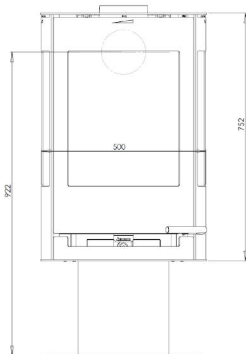
Čelní pohled:
