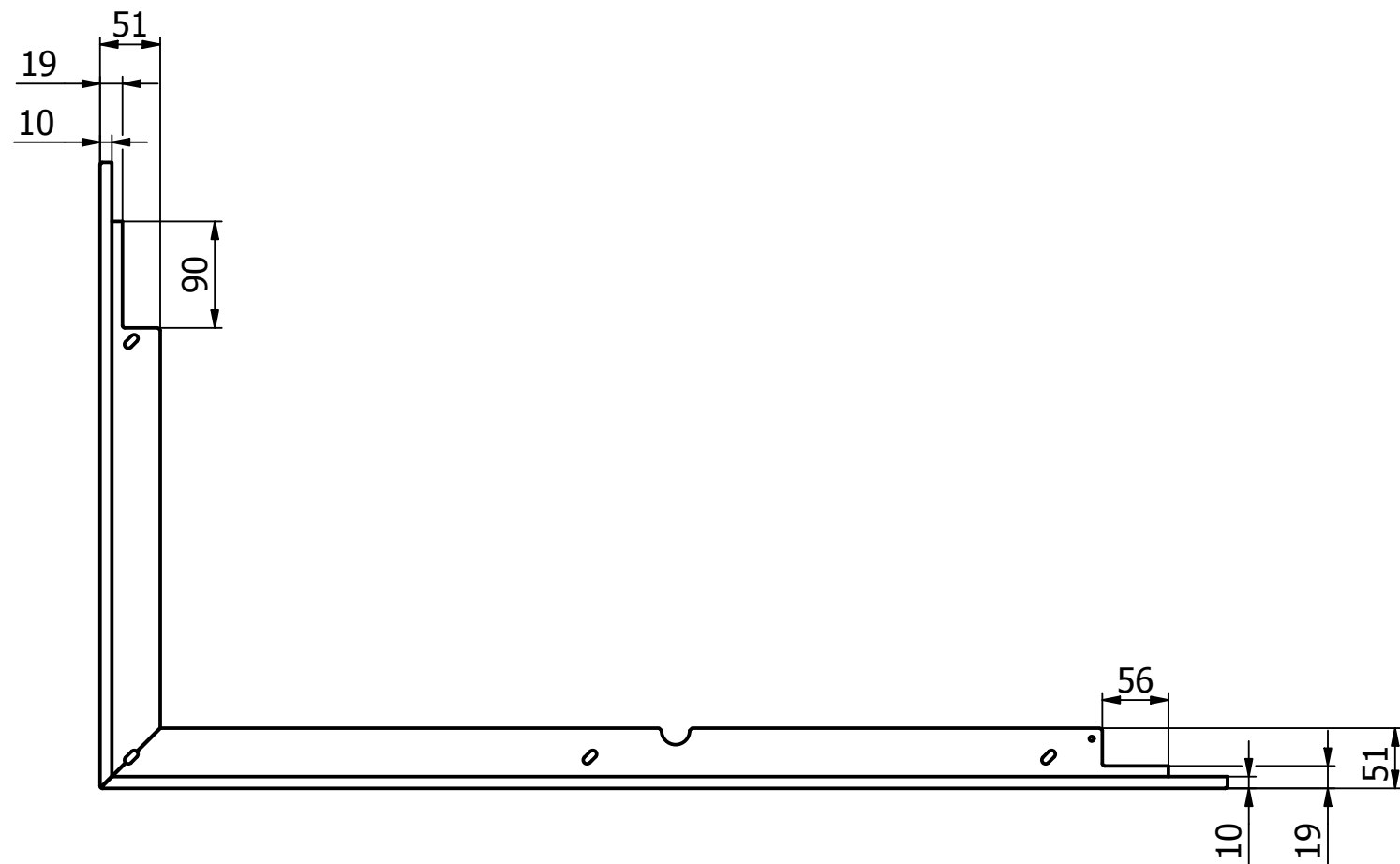
Maskownica 50 płytka
