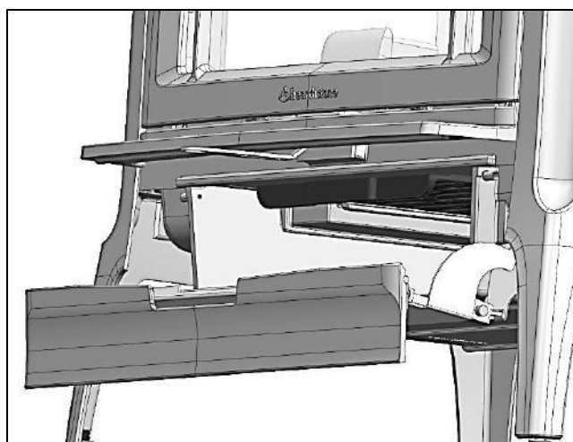
FIG. 5 - Comando agitatore Griglia
