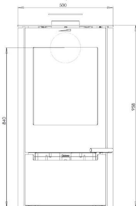
Čelní pohled:
