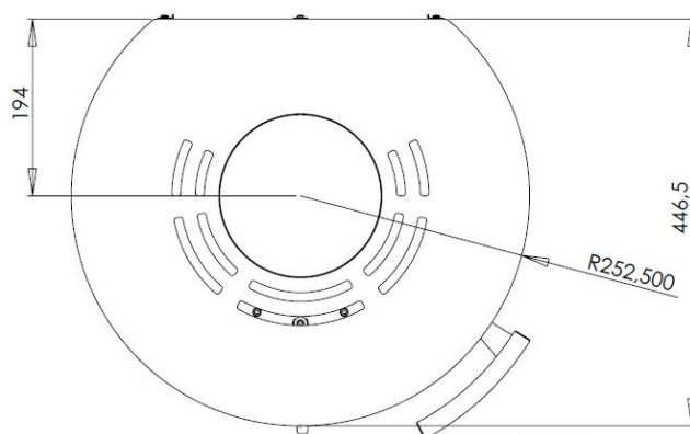
Horní pohled:
