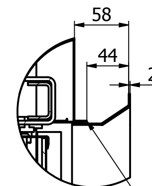
C ( 1 : 4 )
