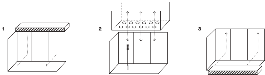
kuva 7 / Lämmönvaihtimen puhdistus
