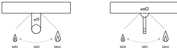
kuva 4 / Ilmansäätövivut
