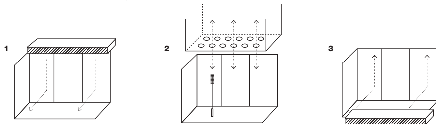
fig. 7 // Pulizia dello scambiatore acqua
