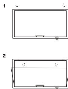
kuva 6 / Luukun avaus puhdistusasentoon
