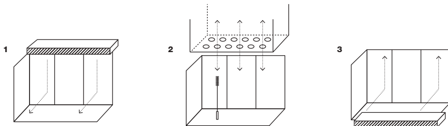
7. kép / vizes hőcserélő tisztítása
