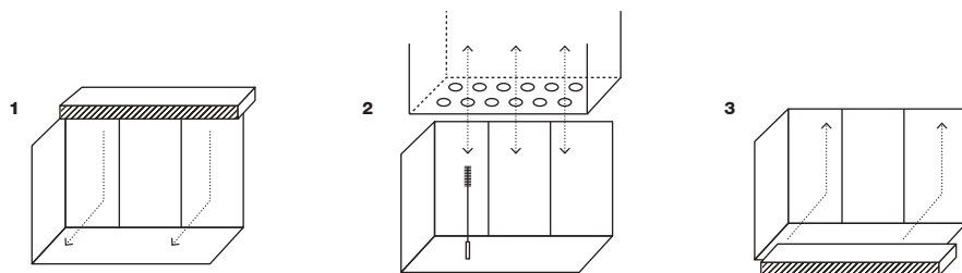
obr. 7 / Čistenie teplovodného výmenníka
