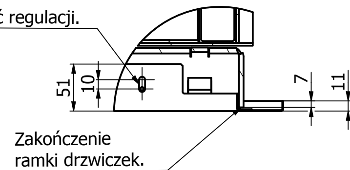
C (1 : 4)
