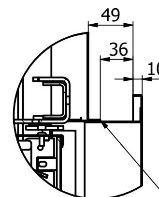
C ( 1 : 4 )
