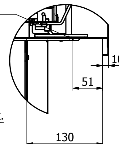
D ( 1 : 4 )
