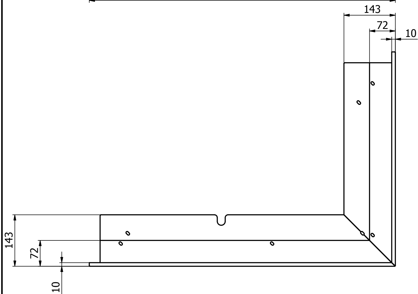
Maskownica 30 głęboka
