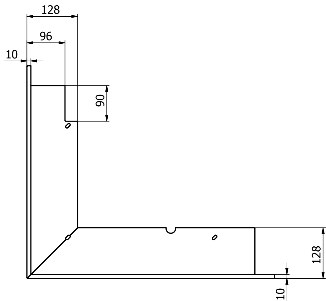
Maskownica 50 głęboka
